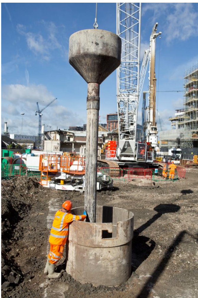
Concrete pour on going
